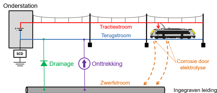
Afbeelding 2.31 - Zwerfstroom en kathodische bescherming
