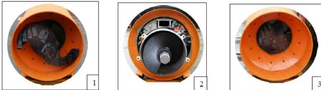
Afbeelding 2.16 - Open boorschild open (1) Afbeelding 2.17 - Achterzijde van microtunnelingsmachine (2) Afbeelding 2.18- Gesloten boorschild (3)
