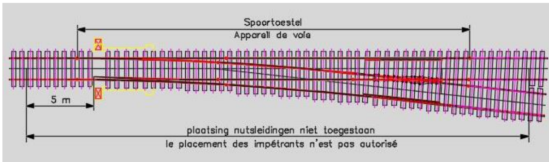
Afbeelding 2.2 - Verboden werkzone - spoorstoel
