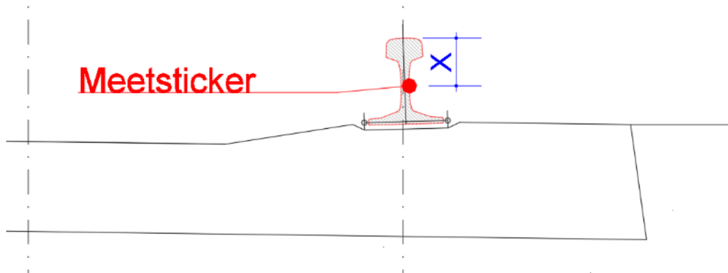
Afbeelding 2.12 - Plaatsing van de meetsticker
