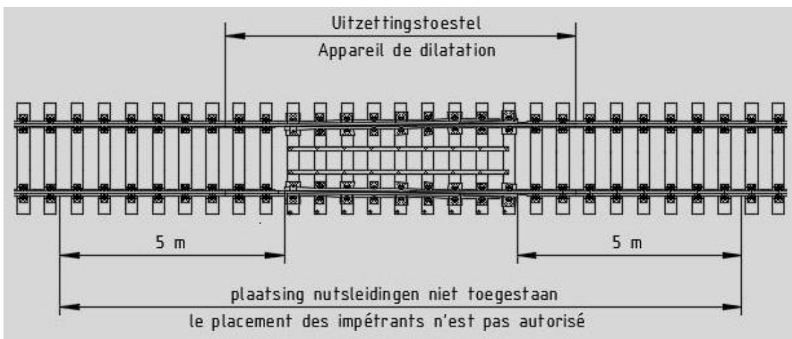
Afbeelding 2.3 - Verboden werkzone - uitzettingstoel
