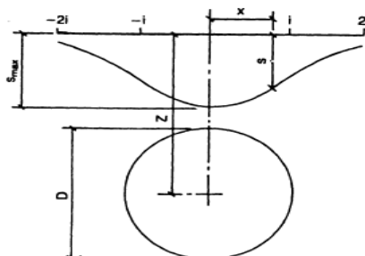
Afbeelding 2.22 - karakteristieken van de waarschijnlijkheidskromme als zettingstrog boven cirkelvormige tunnel
