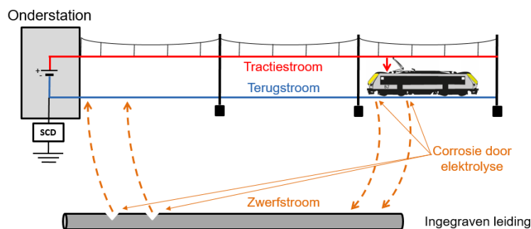
Afbeelding 2.30 - Zwerfstroom en elektrolytische corrosie
