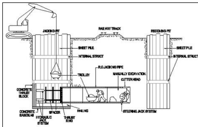
Afbeelding 2.15 – Open front techniek
