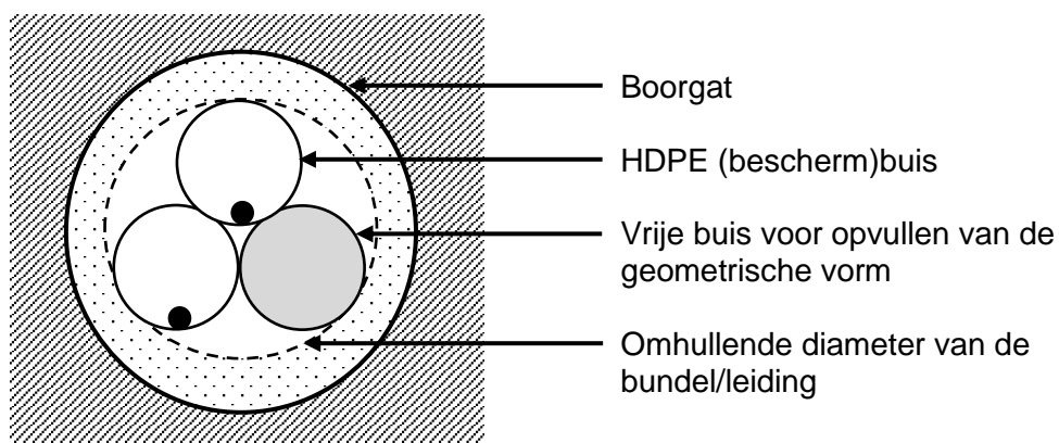
Afbeelding 2.7 – Dwarsdoorsnede gestuurde boring
