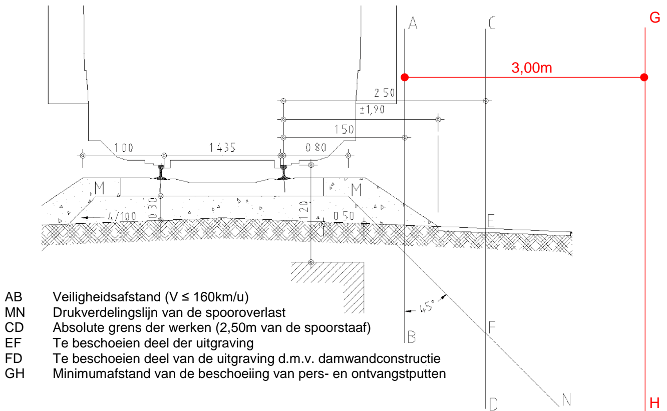
Afbeelding 2.13 - Uitgravingen naast de sporen
