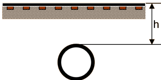
Afbeelding 2.8 - Minimale dekking
