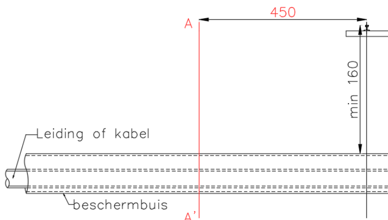
Afbeelding 2.9 - Minimale afstand
