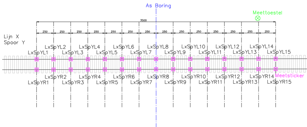
Afbeelding 2.11 - Werkzone bovenaanzicht
